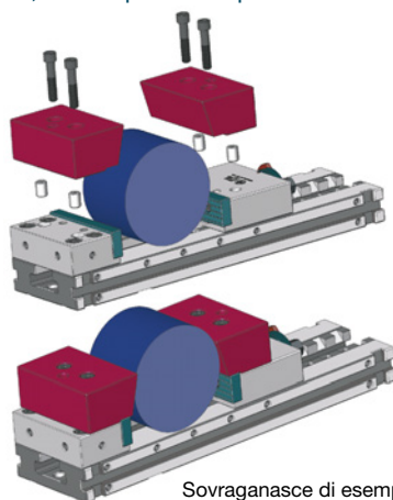
Sovraganasce di esempio Example of top-mounted jaws Exemple de surmachoires
